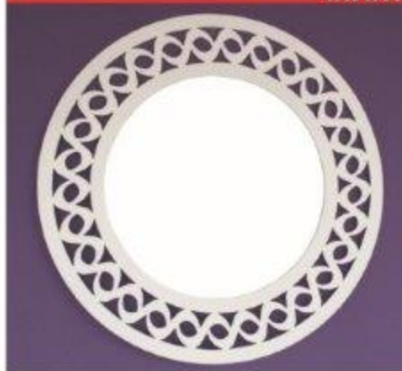
frame рамка 500 x 500 x 3 mm mirror зеркало 420 x 420 x 4 mm sheet metal лист
